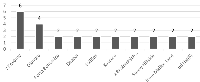
Statistika CHS
